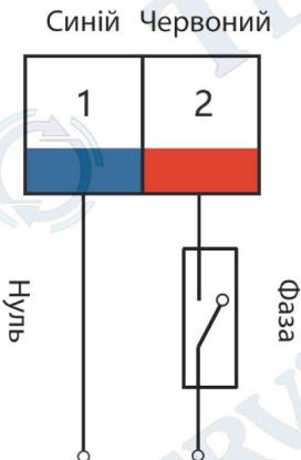
Схема електричного підключення
